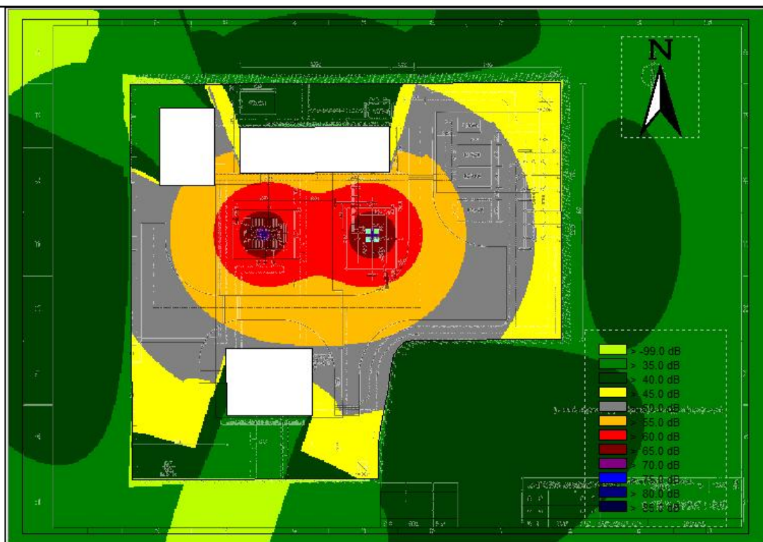
图4-3 黄舟110kV变电站噪声预测等声级线图
