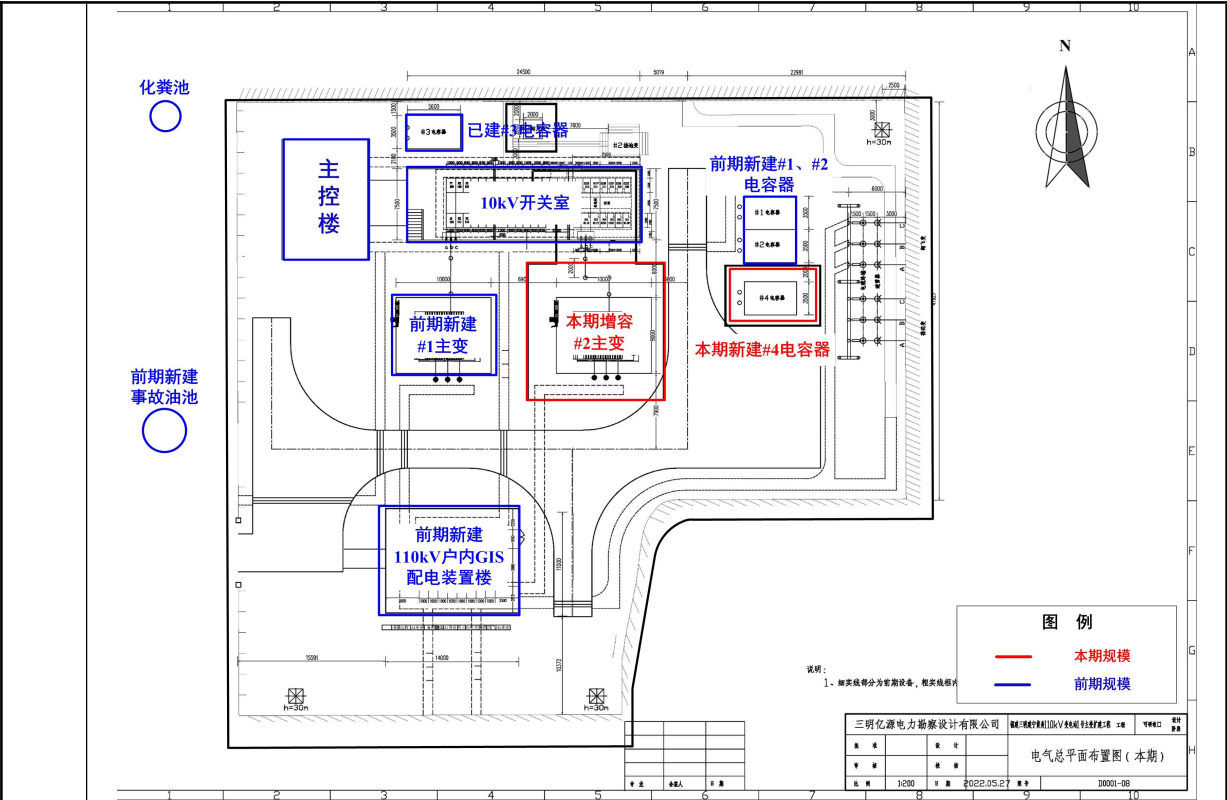
图 2-2 黄湾 110kV 变电站总平面布置图
