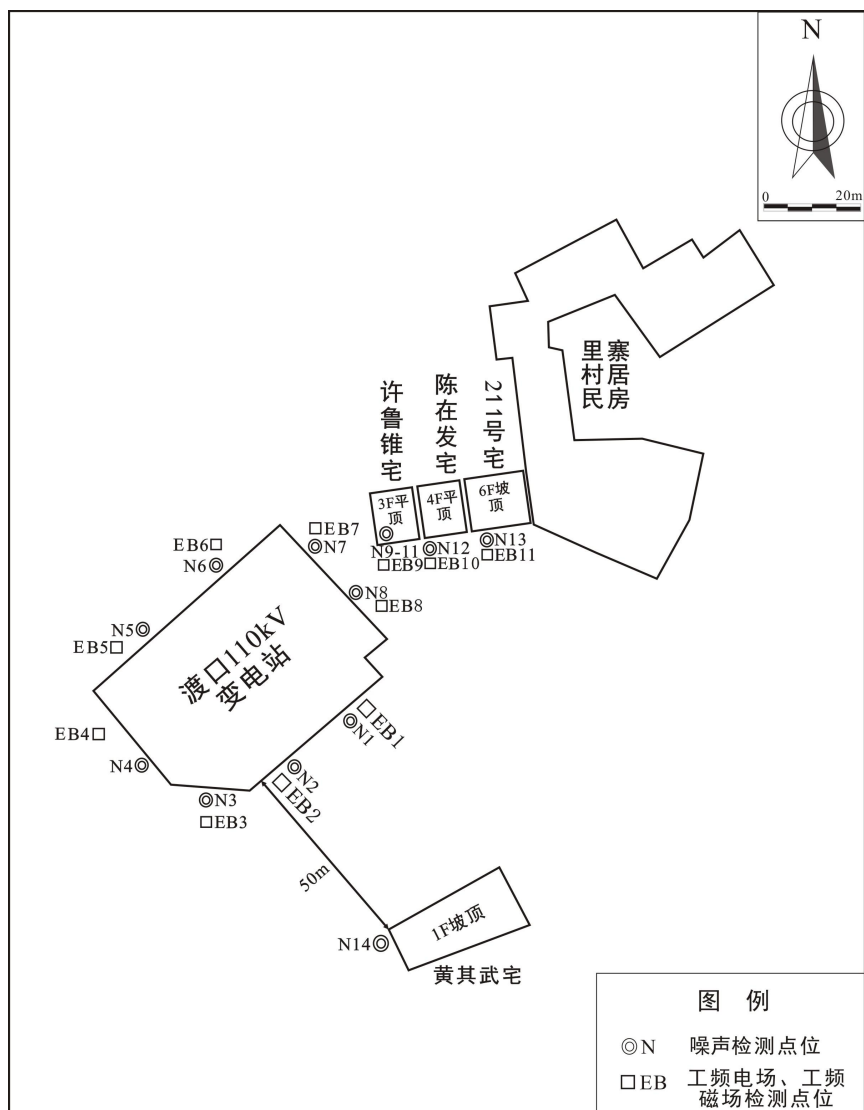
图 A-2 渡口 110kV 变电站平面布置及监测点位图
