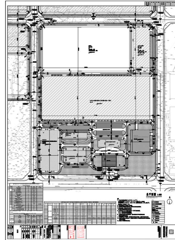
原总平面图
